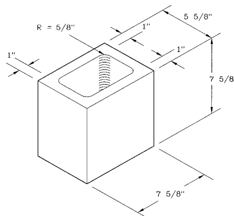
6x8x8 CMU
