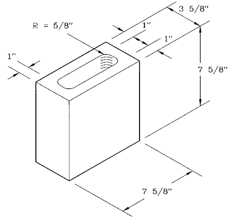
4x8x8 CMU
