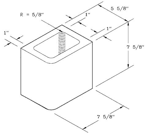
6x8x8 Bullnose CMU
