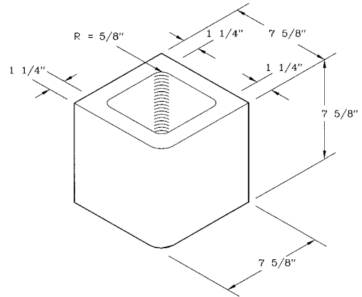
8x8x8 Bullnose CMU
