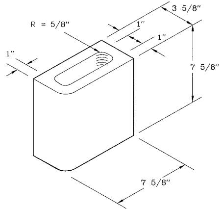
4x8x8 Bullnose CMU
